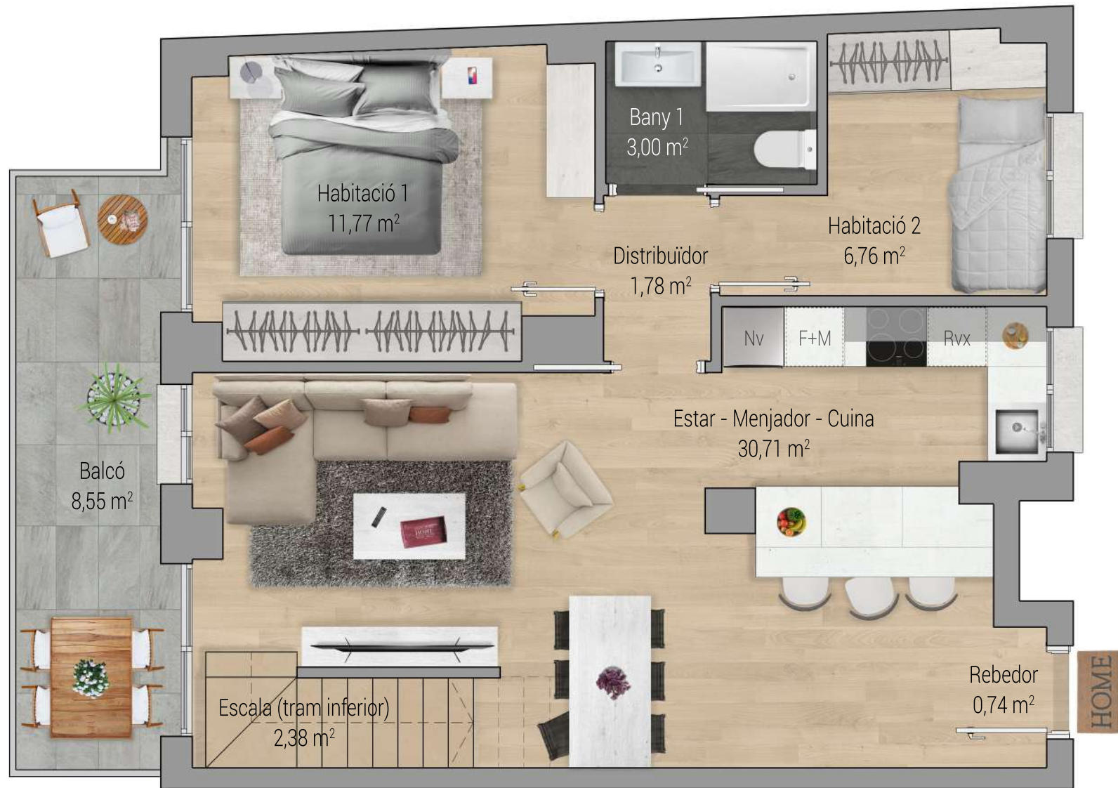
PLANTA INFERIOR
