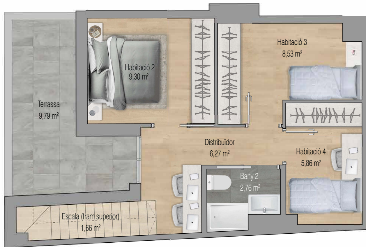
Planta superior
