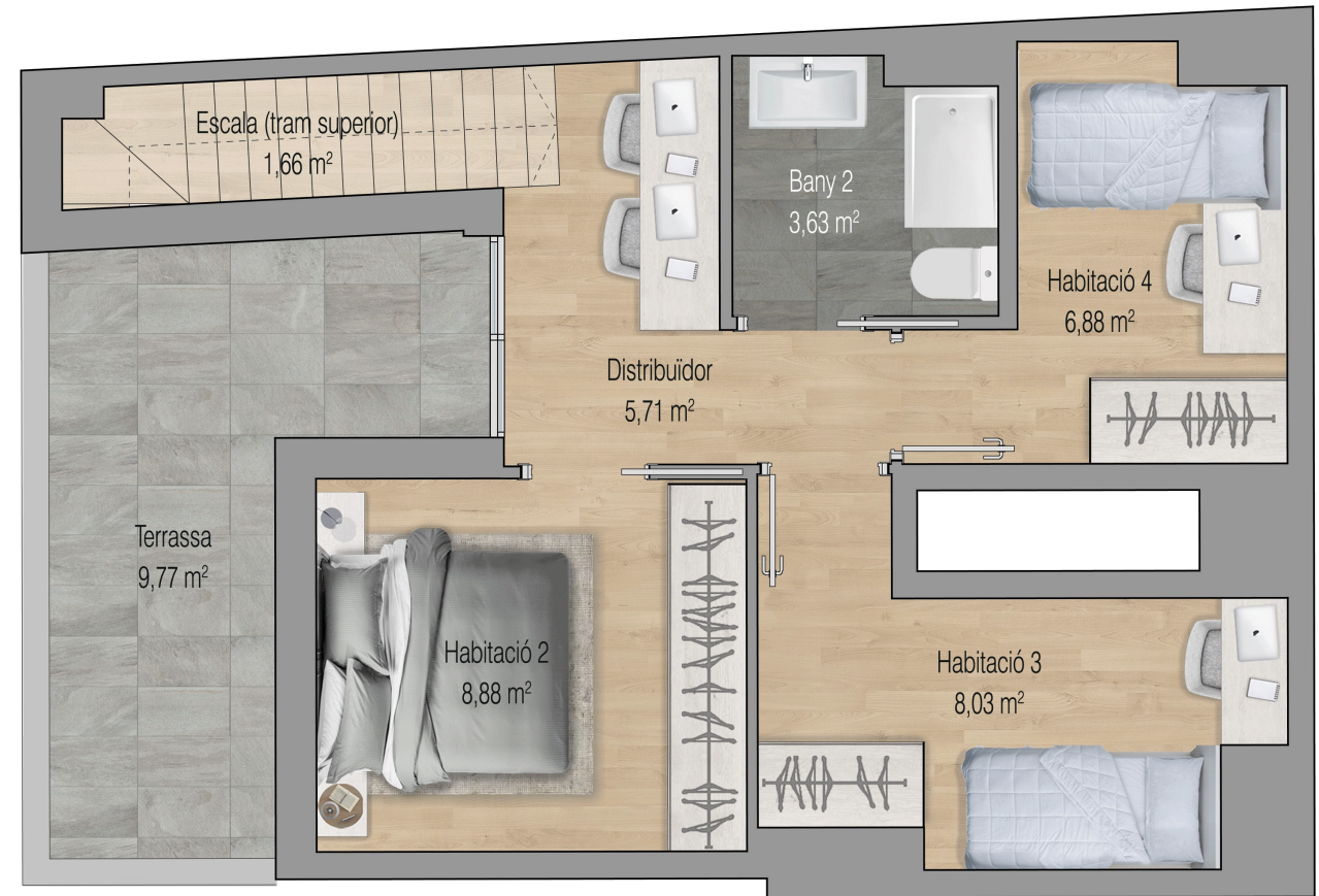
Planta superior
