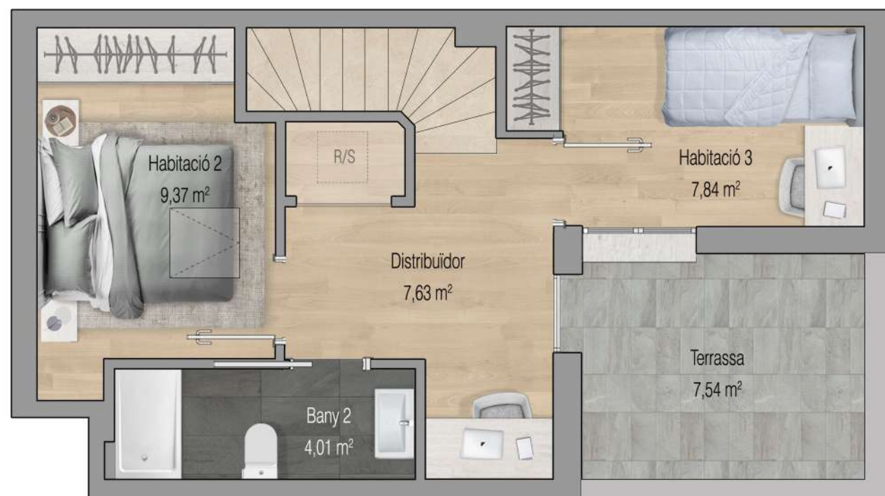
PLANTA SUPERIOR
