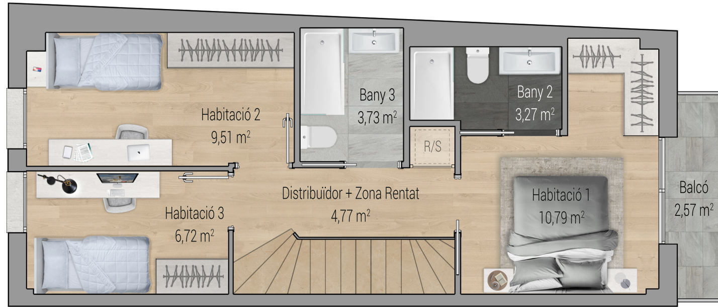
PLANTA PRIMERA
